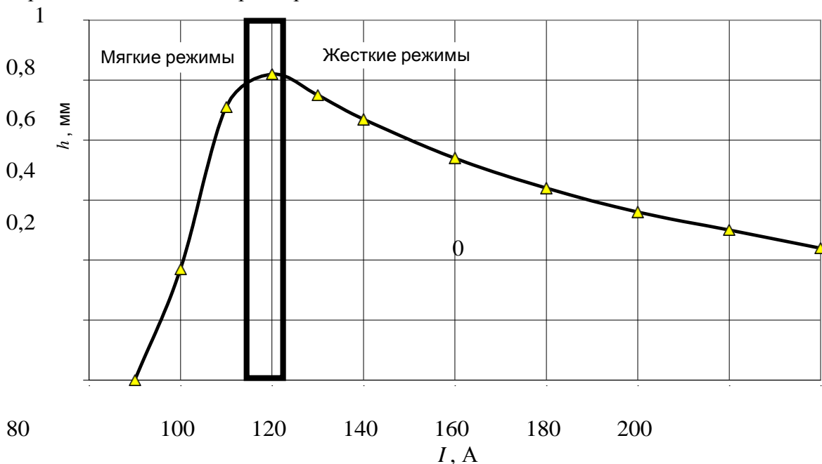
Рис. 2. Зависимость глубины зоны заковки от тока сжатой дуги ( d_{\text{сч}} = 3 мм; s = 20 мм)
